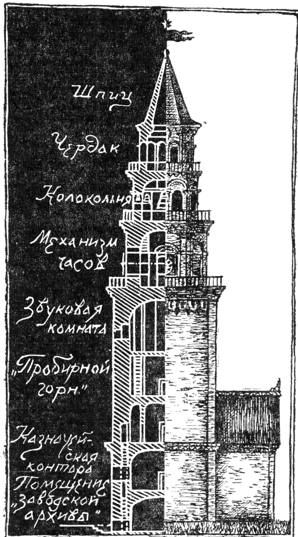
Разрез башни.
